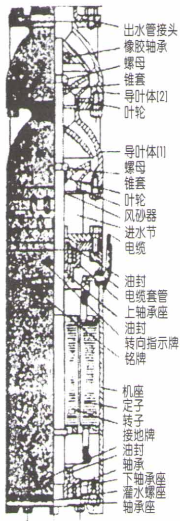
结构原理图
